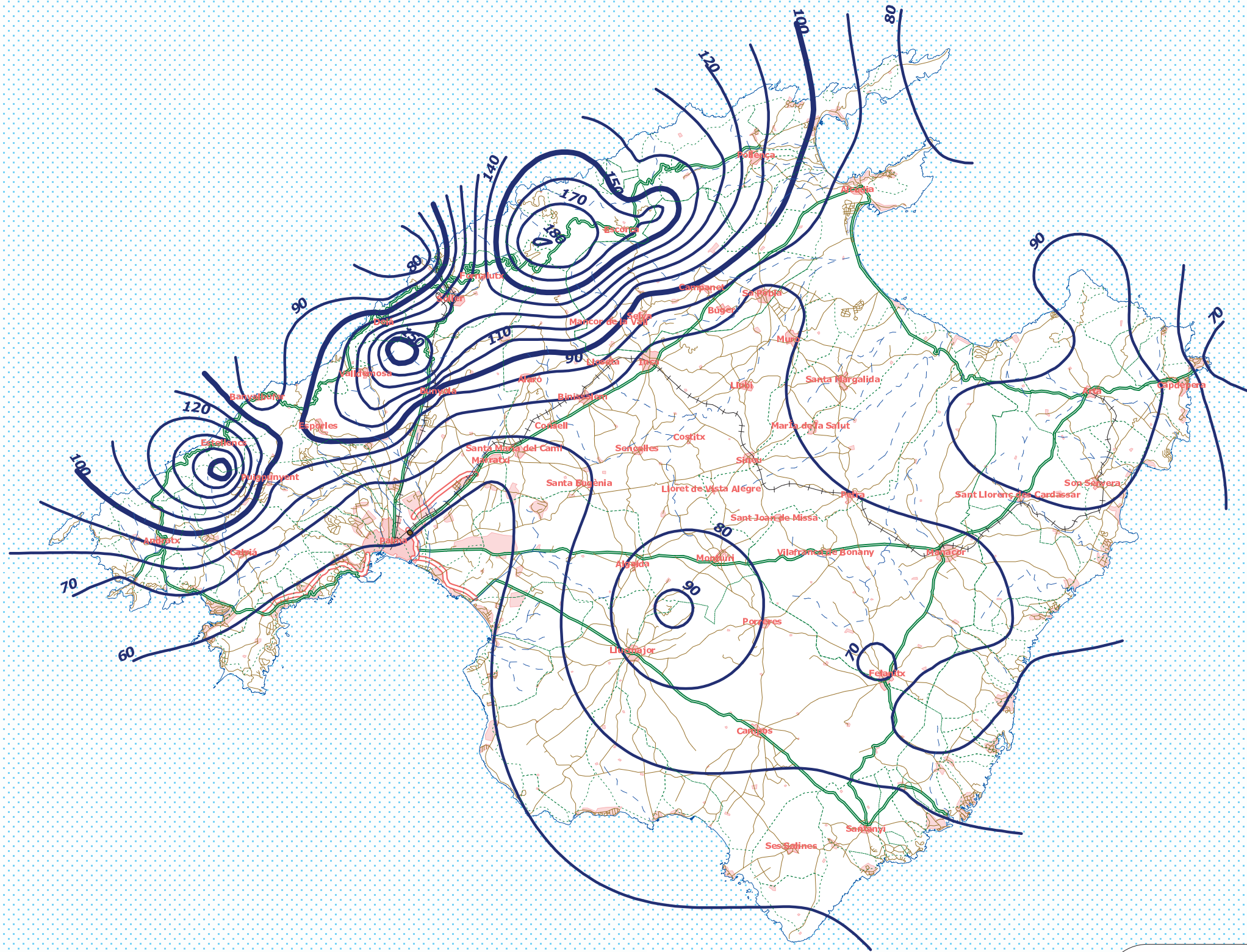
Isla de Mallorca Isohietas máximas diarias (mm) Período de retorno 5 años Escala 1:400.000
