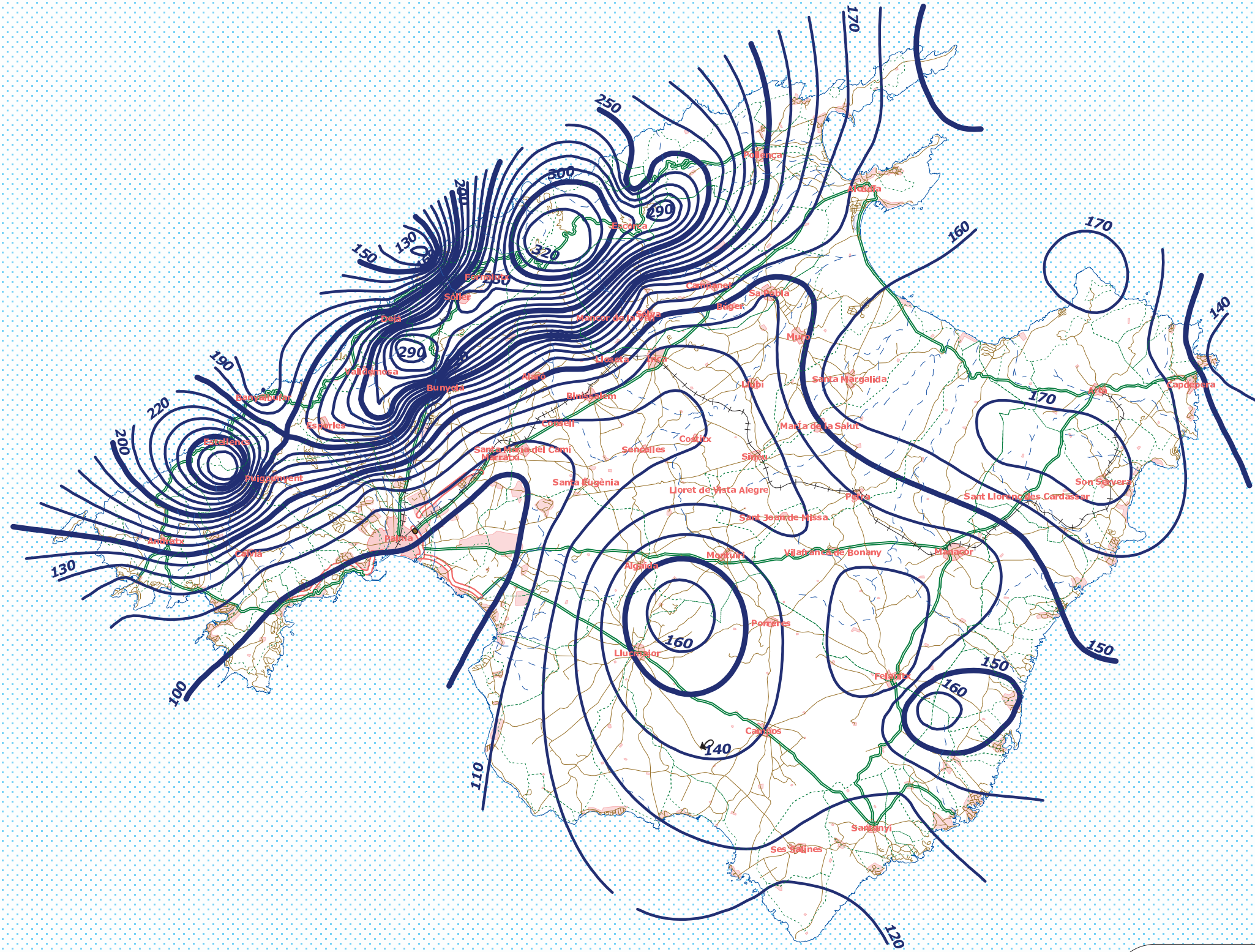
Isla de Mallorca Isohietas máximas diarias (mm) Período de retorno 100 años Escala 1:400.000
