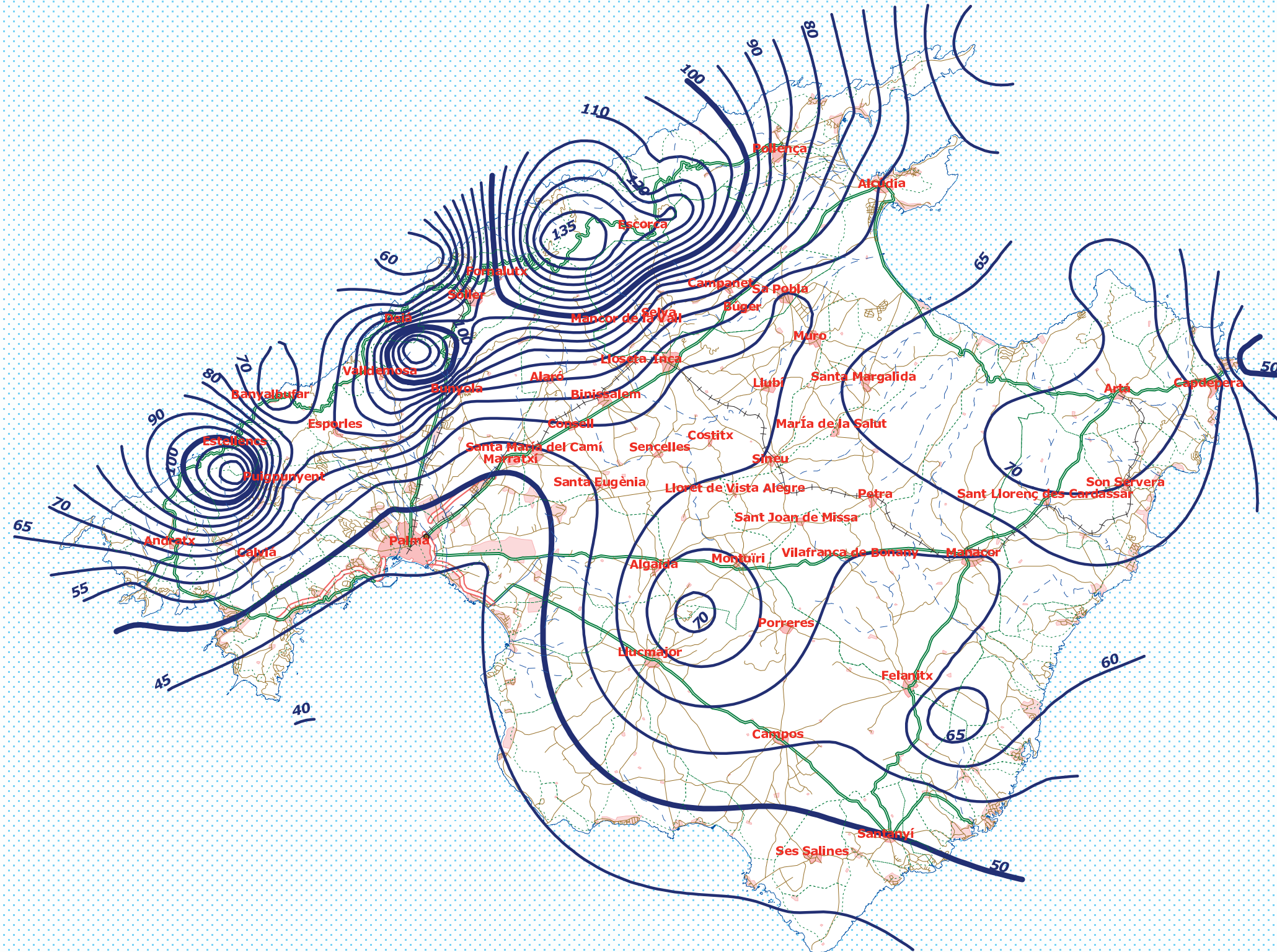
Isla de Mallorca Isohietas máximas diarias (mm) Período de retorno 2.33 años Escala 1:400.000
