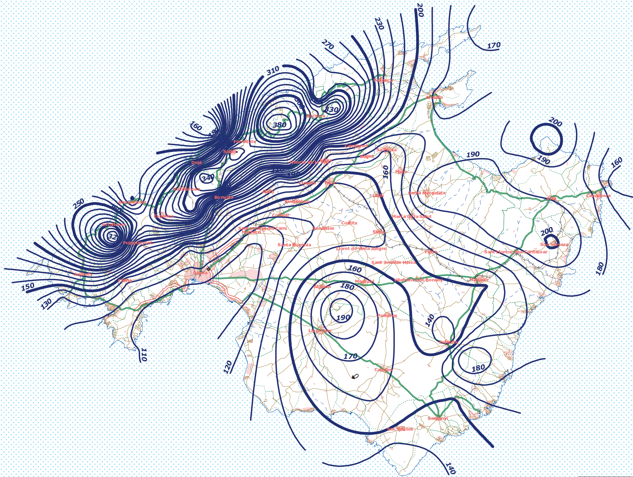
Isla de Mallorca Isohietas máximas diarias (mm) Período de retorno 250 años Escala 1:400.000
