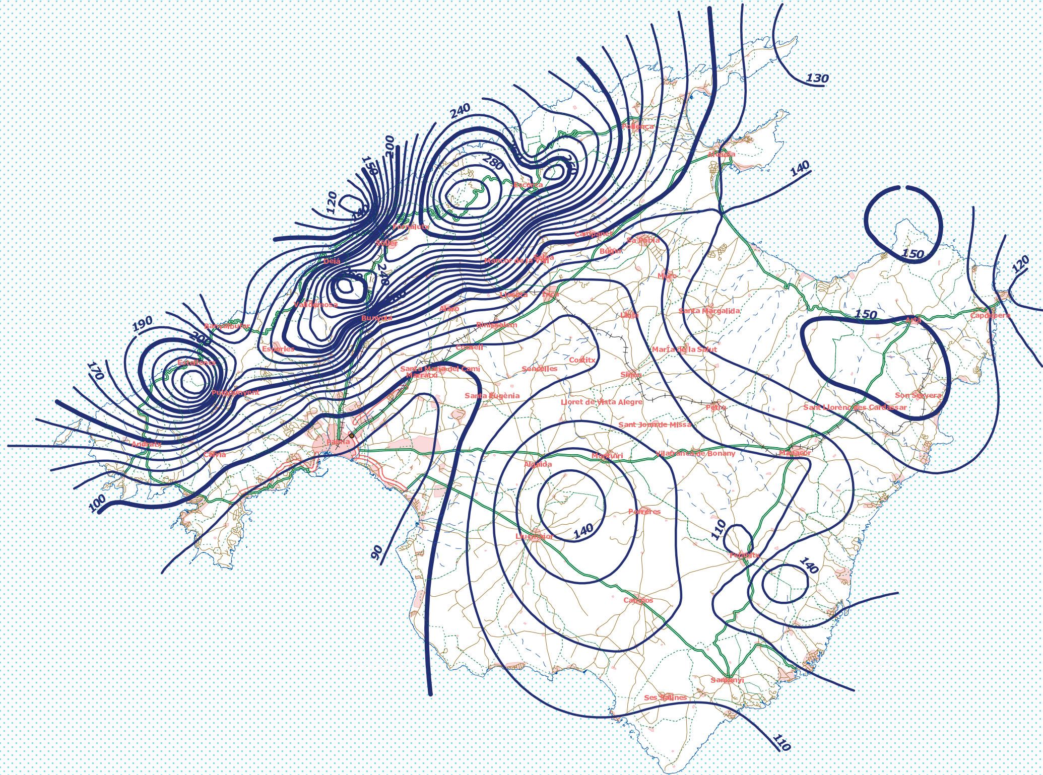
Isla de Mallorca Isohietas máximas diarias (mm) Período de retorno 50 años Escala 1:400.000
